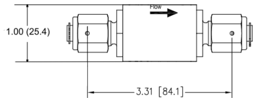
1 : 寸法参考図
