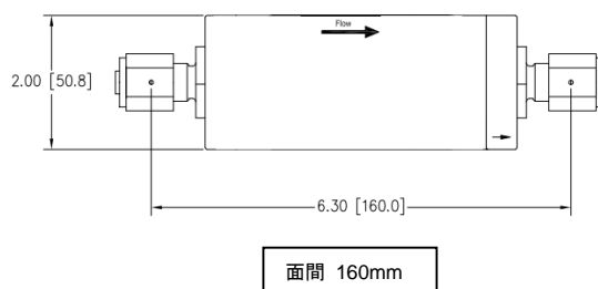
1 : 寸法参考図
